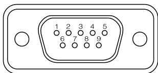
HALL感測器接頭 D-SUB 9PIN 接頭(公)
